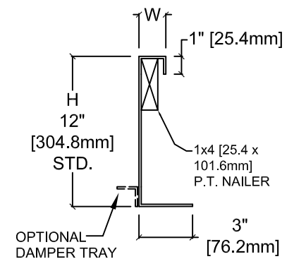
SECTION "A-A" UCC-5
